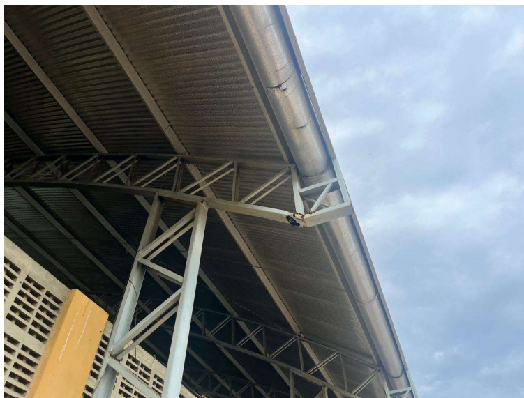
Foto 06 – Imagem externa do ginásio, ponto de oxidação na estrutura metálica, na junção do arco com apoio da calha.
