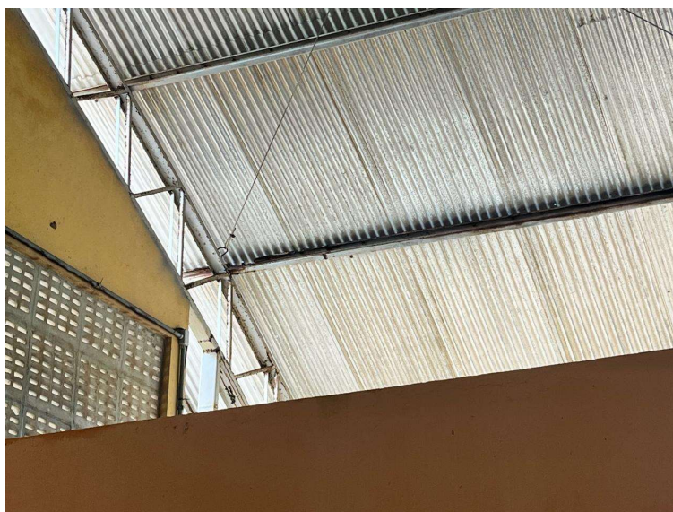
Foto 04 – Imagem interna do ginásio, pontos de oxidação no arco mais externo (viga metálica da fachada frontal) da estrutura metálica do ginásio.
