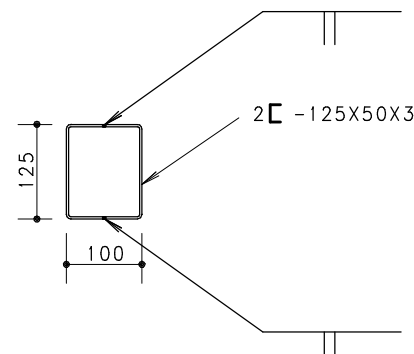
SEÇÃO 1-1
