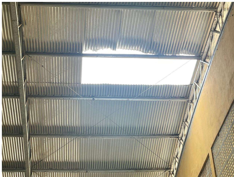
Foto 01 – Imagem interna do ginásio, com ausência de telha de alumínio e telha danificada, próximo a face da fachada frontal.
