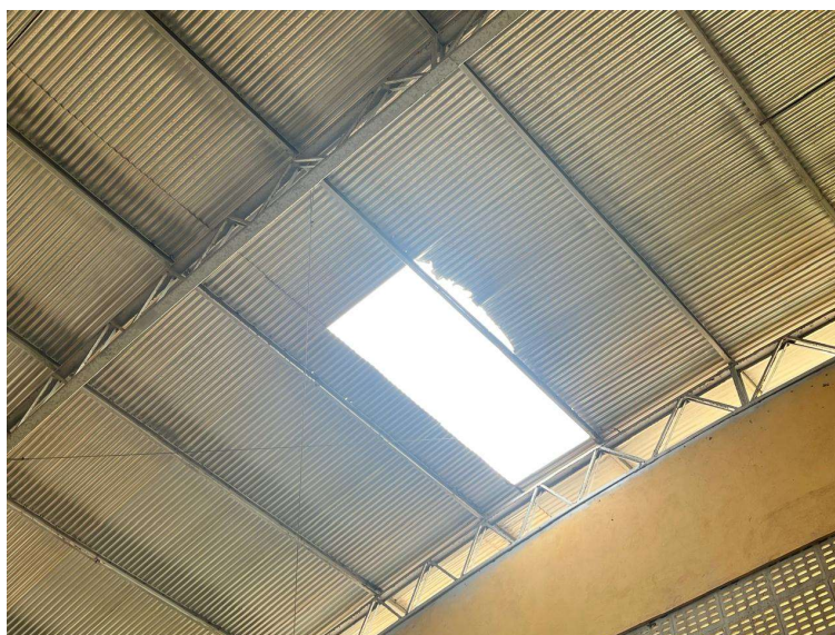
Foto 02 – Imagem interna do ginásio, com ausência de telha de alumínio e telha danificada, próximo a face da fachada frontal.
