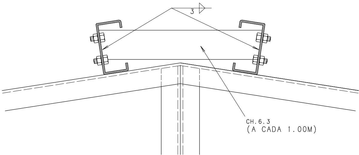
DETALHE 5 REFORÇO NAS TERÇAS DA CUMEIRA
