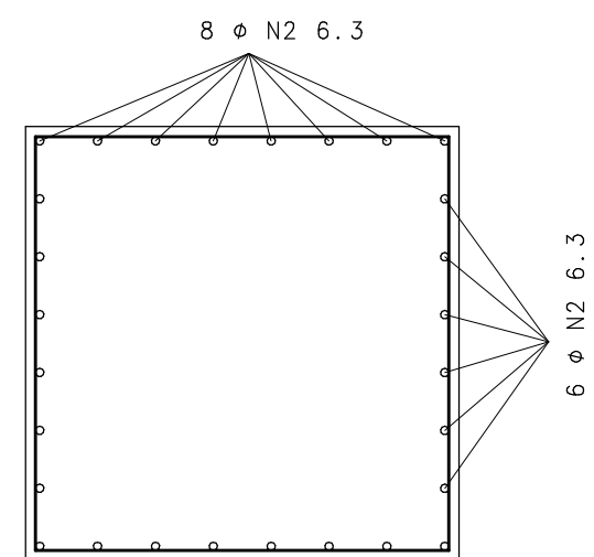
ARMAÇÃO DA SAPATA
