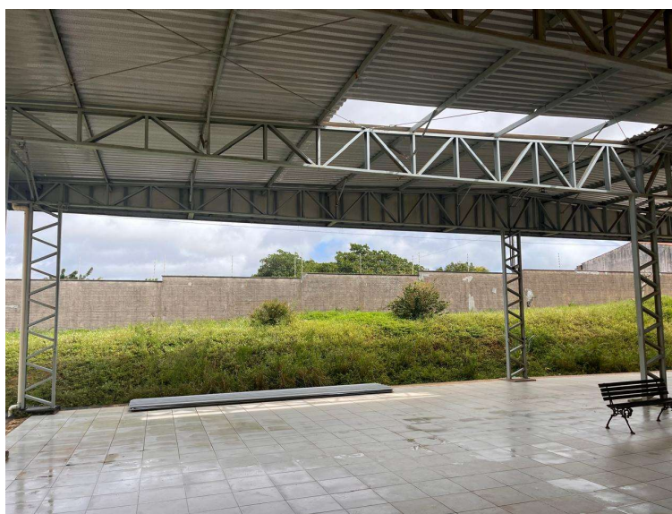
Foto 16 – Área de vivência, um dos locais que está sem a telha de alumínio (Final da Foto 13).
