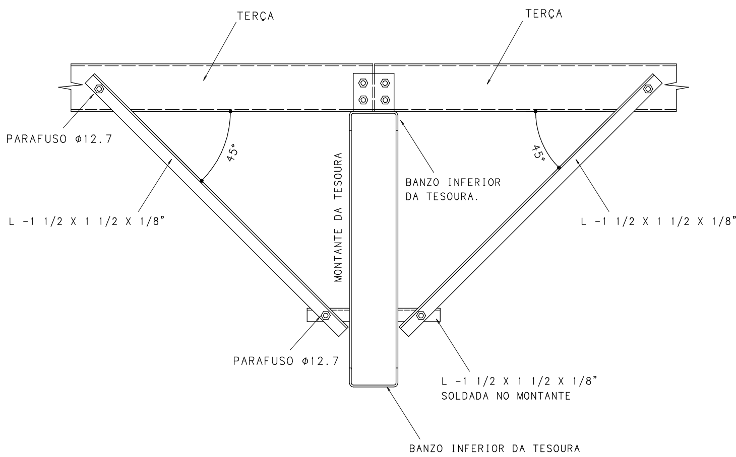
DETALHE 6 CONTRAVENTAMENTO DO BANZO INFERIOR DA TESOURA
