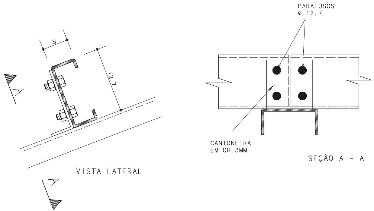
DETALHE 4 LIGAÇÃO TERÇA/TESOURA
