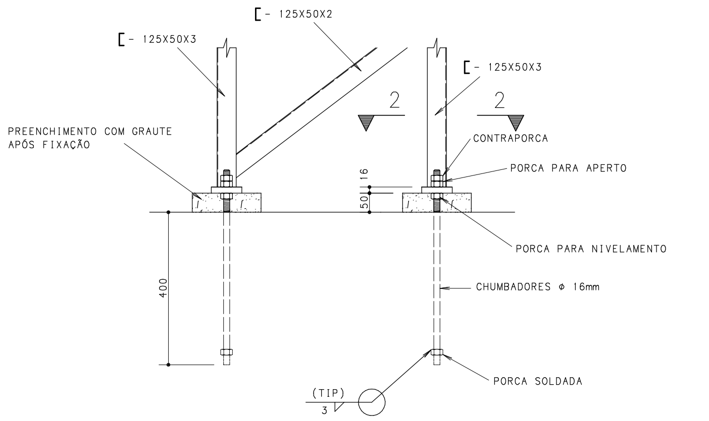
DETALHE 3 ESC. 1:10 LIGAÇÃO DA ESTRUTURA METÁLICA COM AS FUNDAÇÕES 27X
