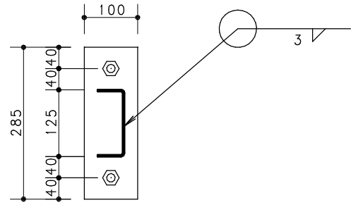
SEÇÃO 2-2 CHAPA DE BASE 100X285X16mm
