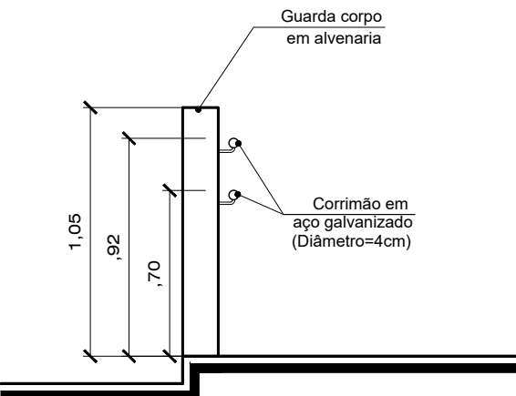
DETALHE 01 Escala: 1/25
