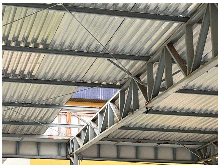
Foto 18 – Área de vivência, oxidação em vigas metálicas.
