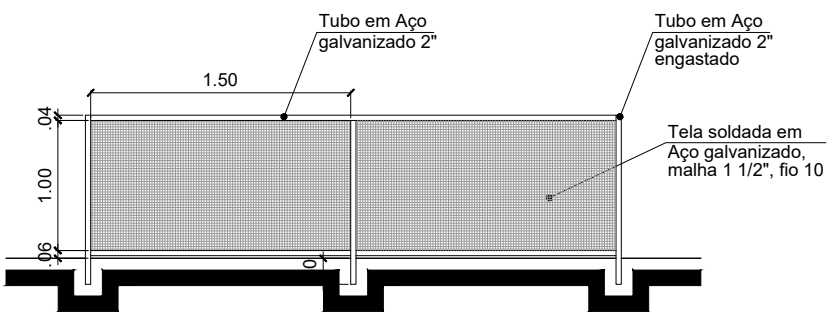
DETALHE 02 Escala: 1/100
