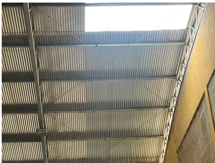
Foto 03 – Imagem interna do ginásio, com ausência de telha de alumínio e telha danificada, próximo a face da fachada frontal.
