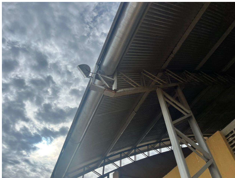
Foto 07 – Imagem externa do ginásio, ponto de oxidação na estrutura metálica.
