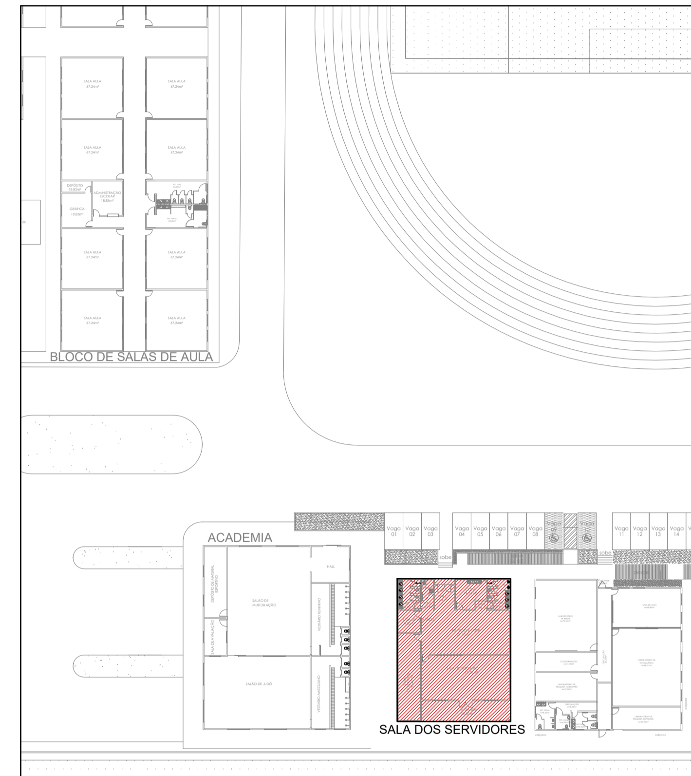
IMPLANTAÇÃO esc: 1/500
