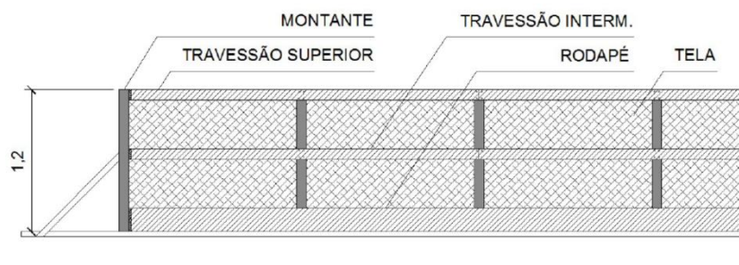
Figura 1 – Detalhe guarda-corpo
