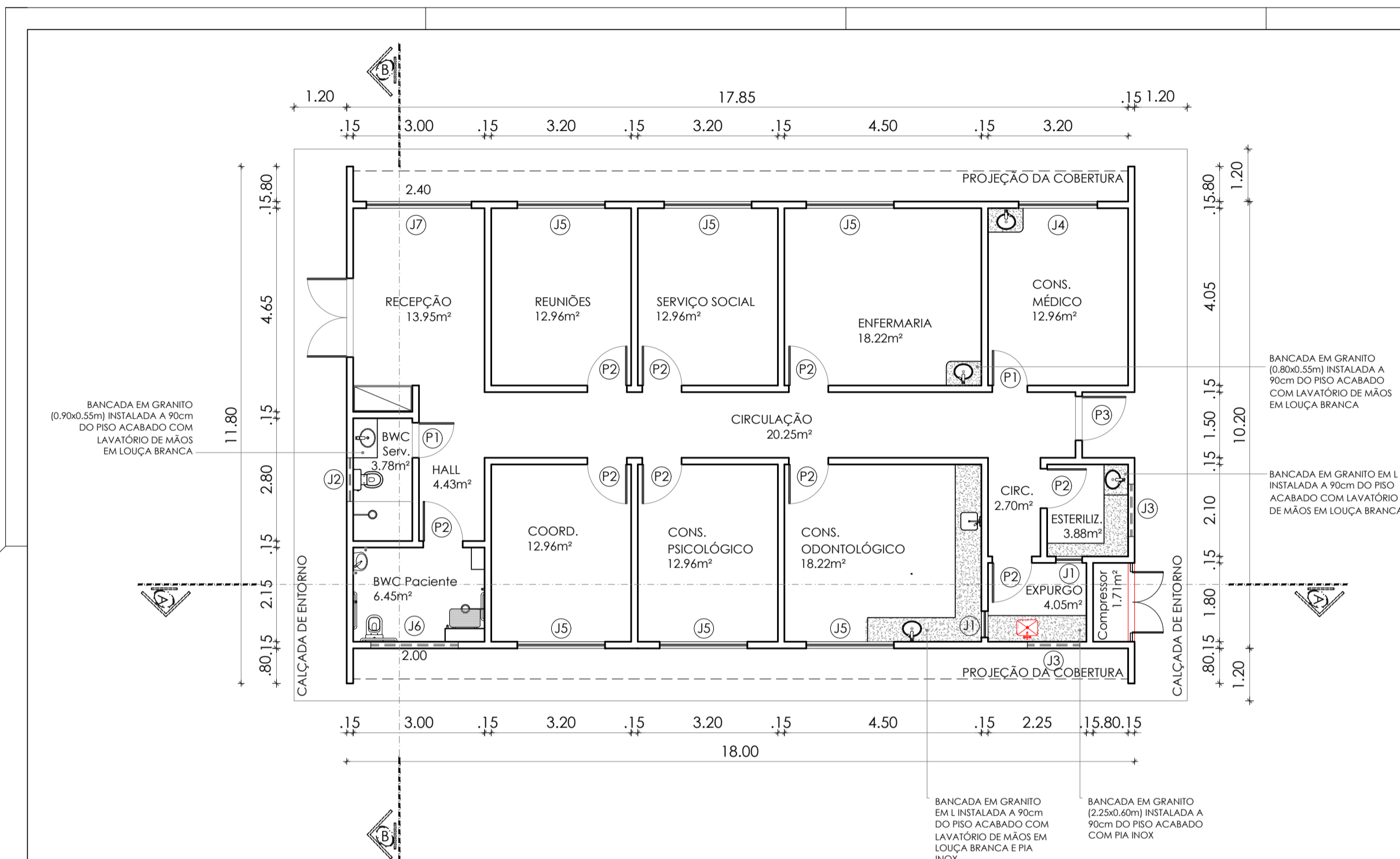
PLANTA BAIXA - SETOR MÉDICO (A CONSTRUIR) ESCALA 1/100
