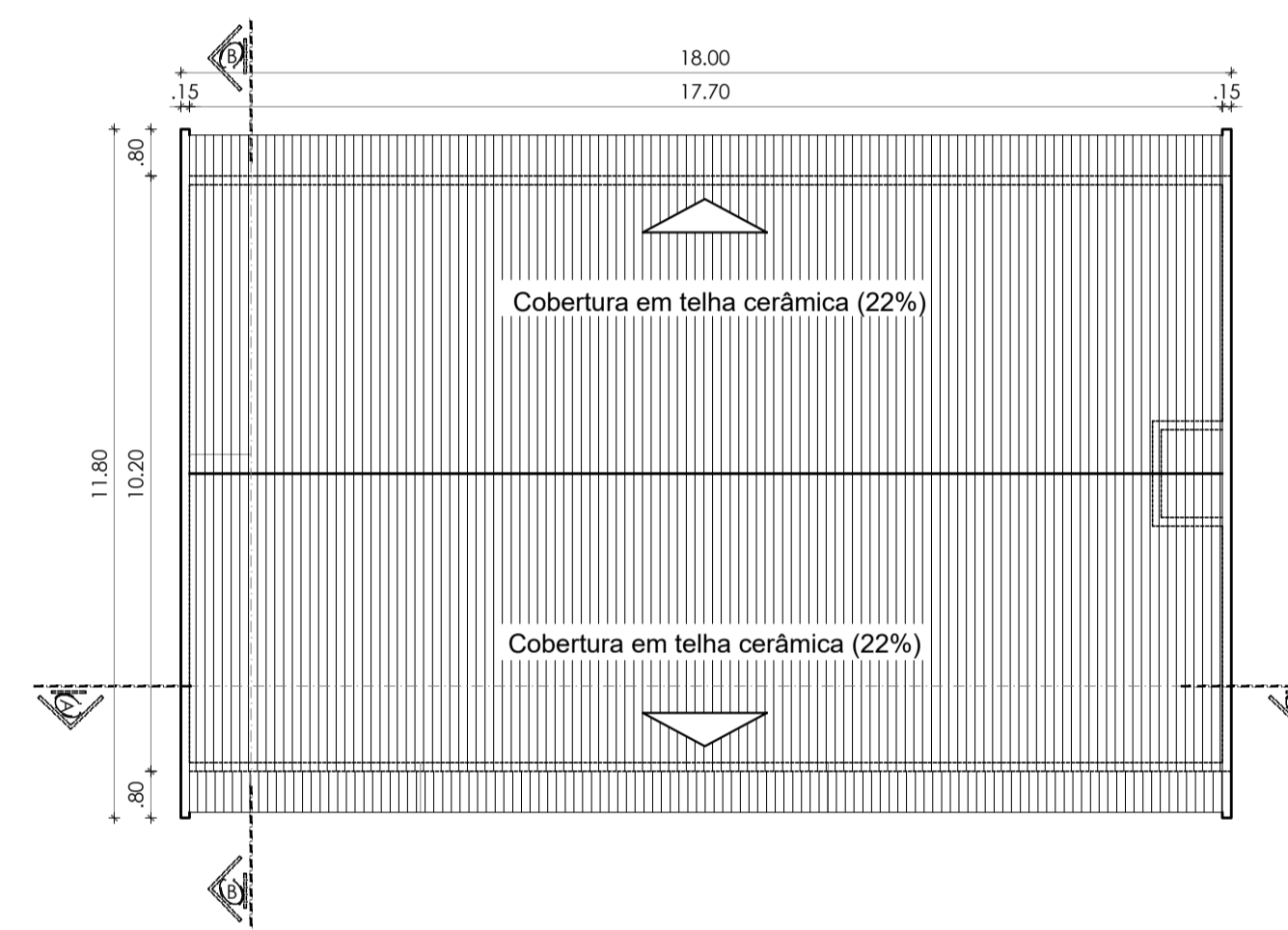
PLANTA DE COBERTURA - SETOR MÉDICO (A CONSTRUIR) ESCALA 1/125
