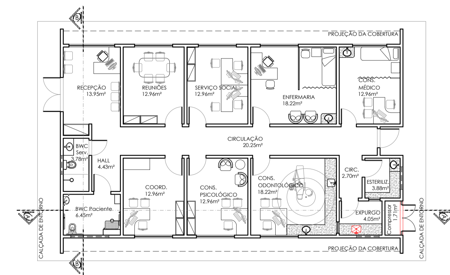
PLANTA DE LAYOUT - SETOR MÉDICO (A CONSTRUIR) ESCALA 1/125
